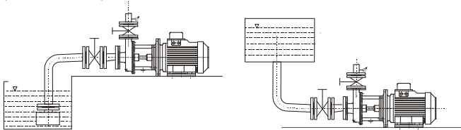
Bild 2 Rohrleitungsanschluss
