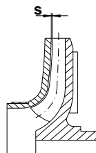
Bild 5: HG Pumpe
